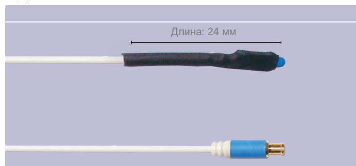
ST100S - Сенсорный зонд с коротким круглым наконечником
