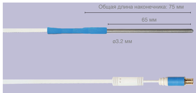
ST100KF - Датчик температуры с плоским кабелем
