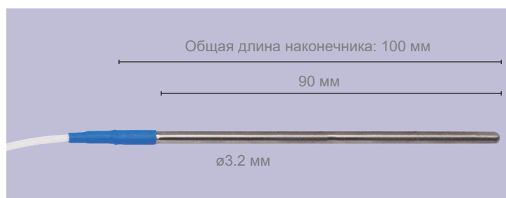
ST100L - Зонд с длинным наконечником
