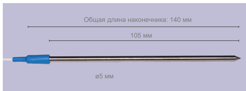
ST100T - Сенсорный зонд с длинным наконечником
